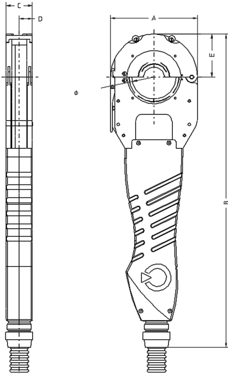
MW 40 varustetaan putkikoon mukaisella Titaani-istukalla (TCI)
