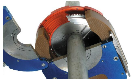
MW 40 varustetaan putkikoon mukaisella Titaani-istukalla (TCI)
